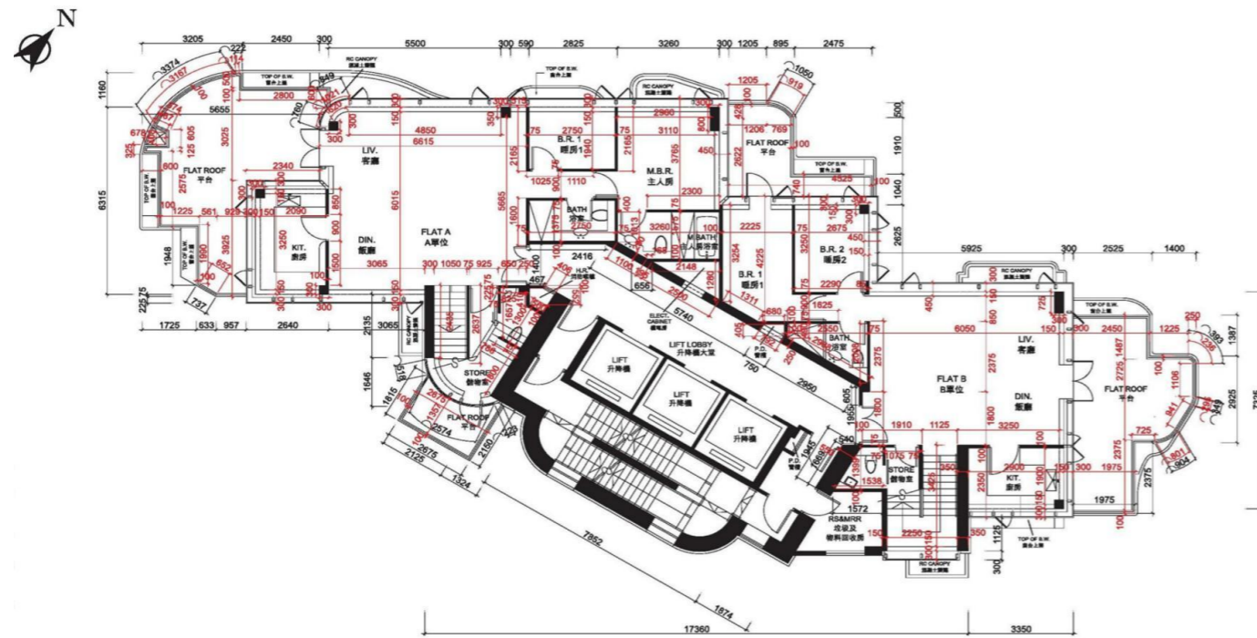
53樓樓面平面圖 53/F FLOOR PLAN
