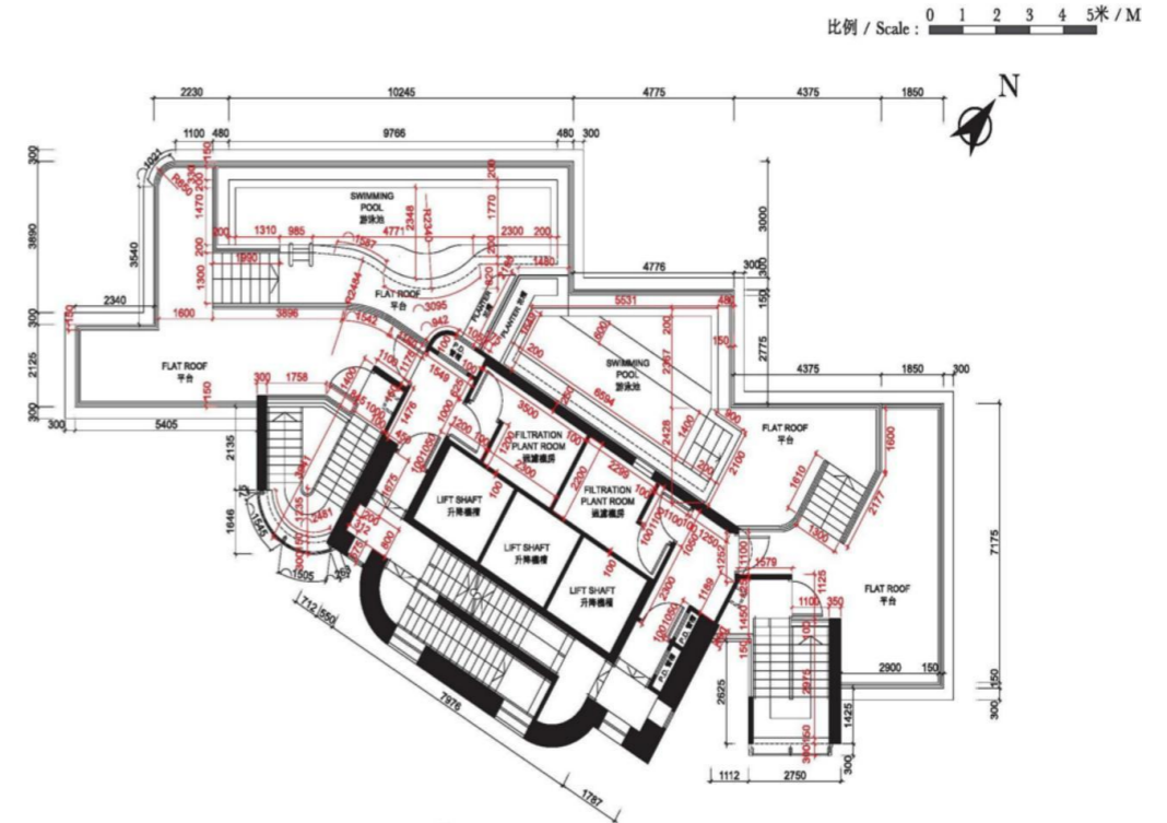
天台樓面平面圖 ROOF PLAN
